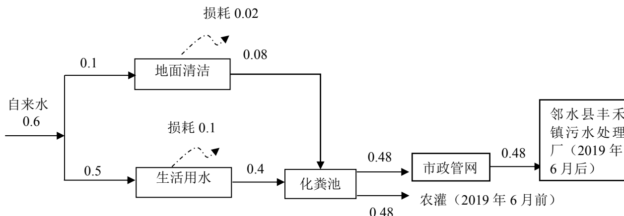
图 2-1 项目水量平衡见图 (m 3 /d)
