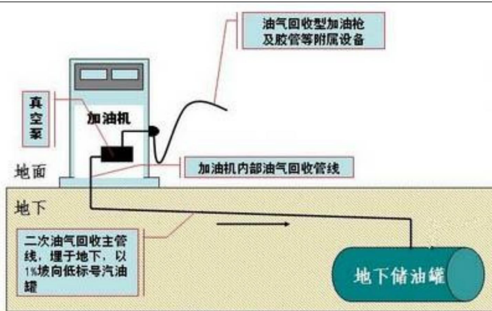
图 2-4 加油油气回收系统示意图
