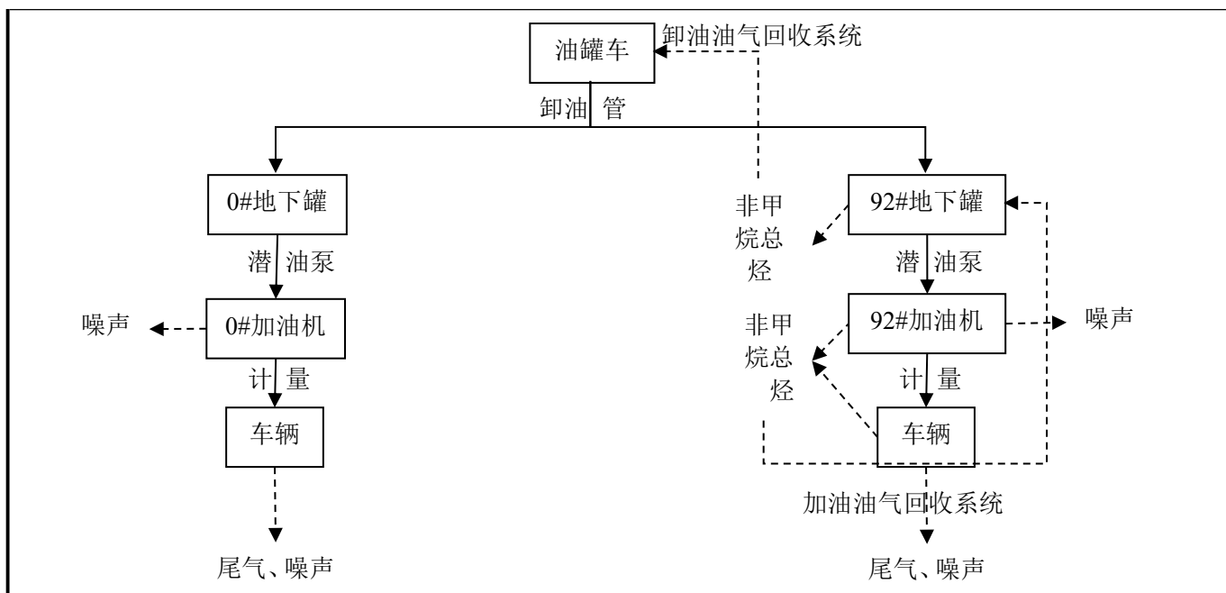
图 2-2 项目运营期工艺流程和产污环节图
