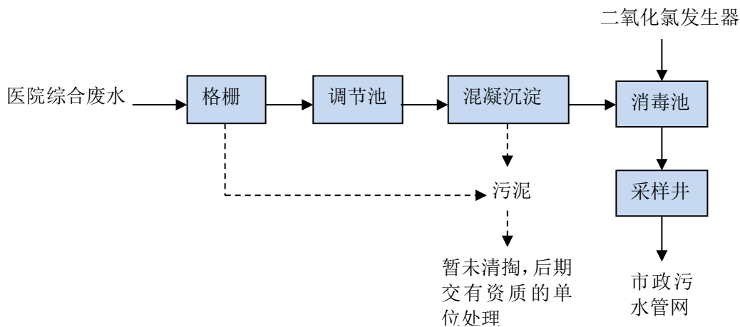
图 3-1 污水处理工艺流程
